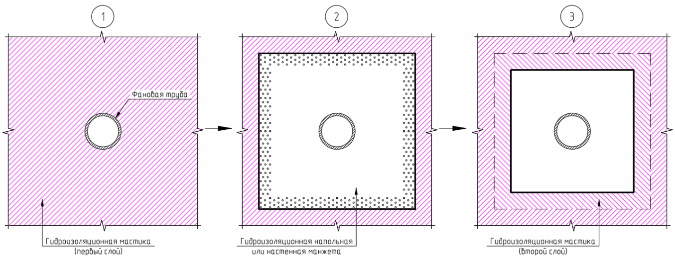
Последовательность нанесения гидроизоляционной манжеты.
